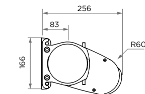
Ambre & Ambre Lux - Pose face -
