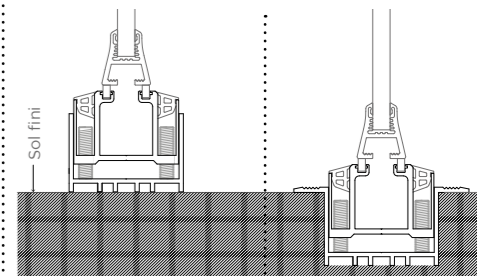
Rail posé au sol standard
