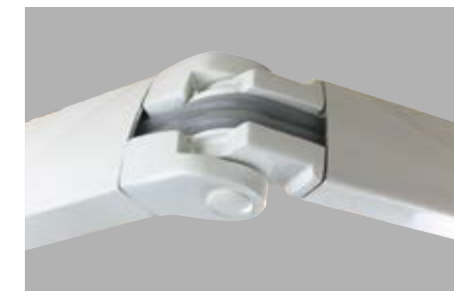
Bras en aluminium thermolaqué munie d'un double câble gainé. Les bras sont testé à 20 000 cycles.
