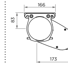
Ambre & Ambre Lux - Pose plafond -
