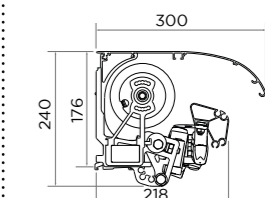
Perle et Perle Lux Pose Face avec auvent
