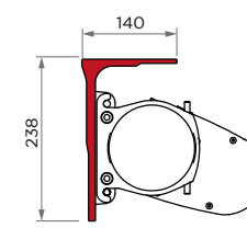
Ambre & Ambre Lux - Pose plafond avec equerre - 27
