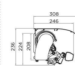
Jade avec auvent Pose Face
